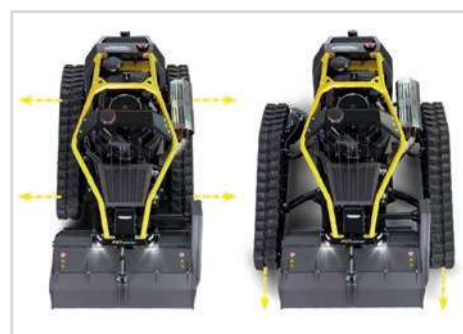
SISTEMA DE ELEVAÇÃO PATENTEADO com variação do centro de gravidade da máquina
